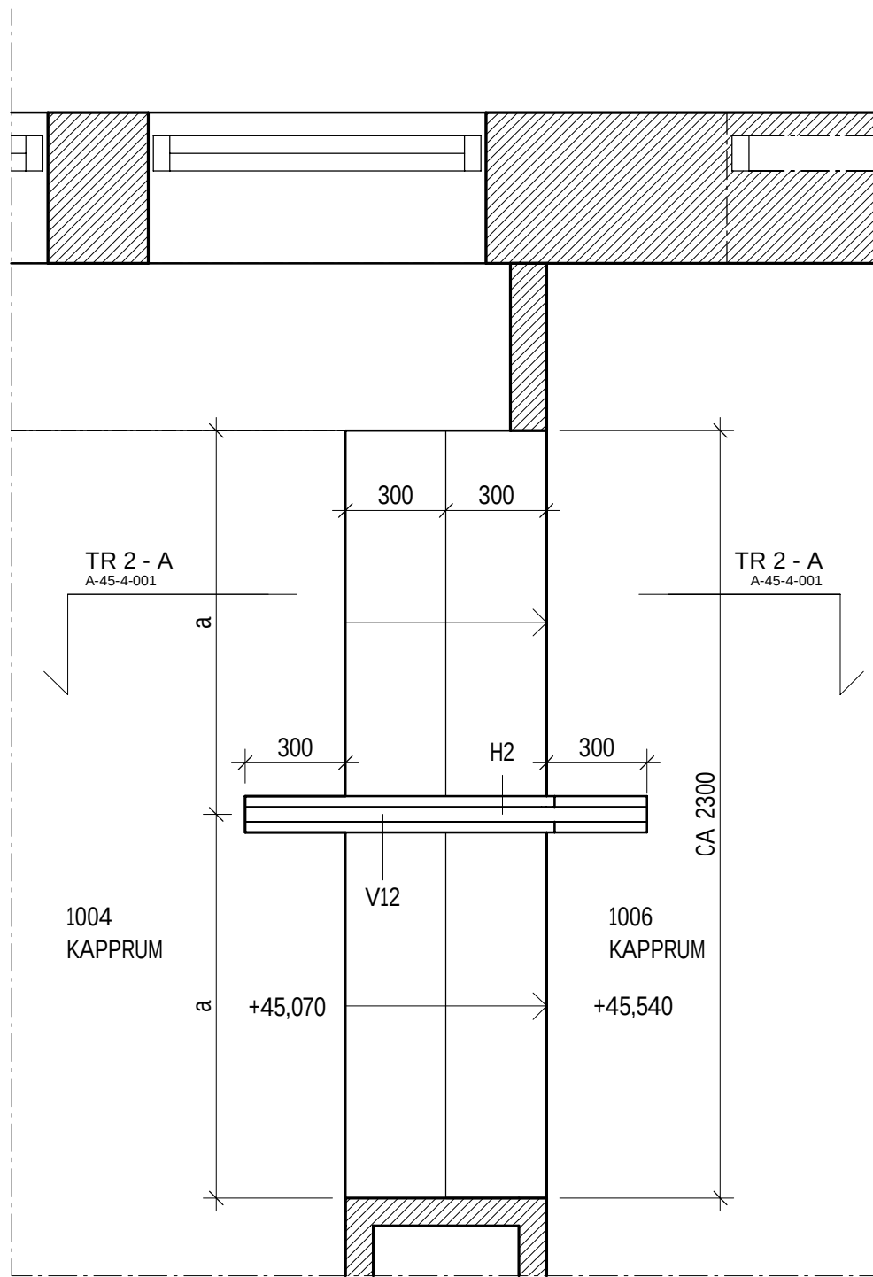
TRAPPA 2 - PLAN 1 : 20
