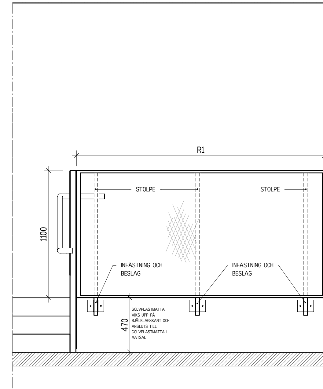
ELEVATION 1 - RÄCKE TYP R1 1 : 20
