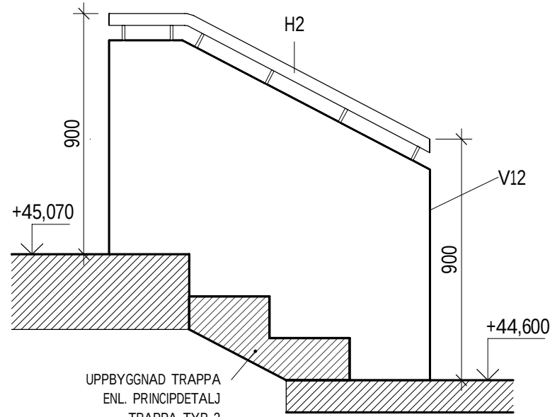
TRAPPA 1 - SEKTION A 1 : 20
