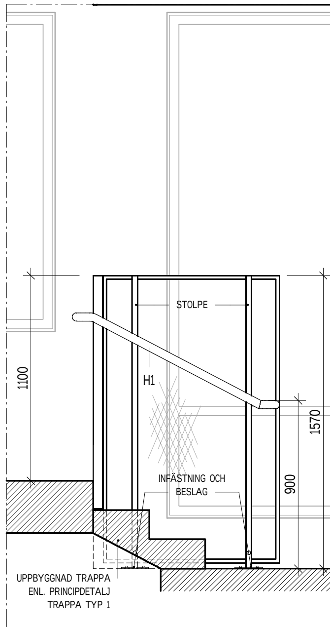
TRAPPA 3 - SEKTION A 1 : 20
