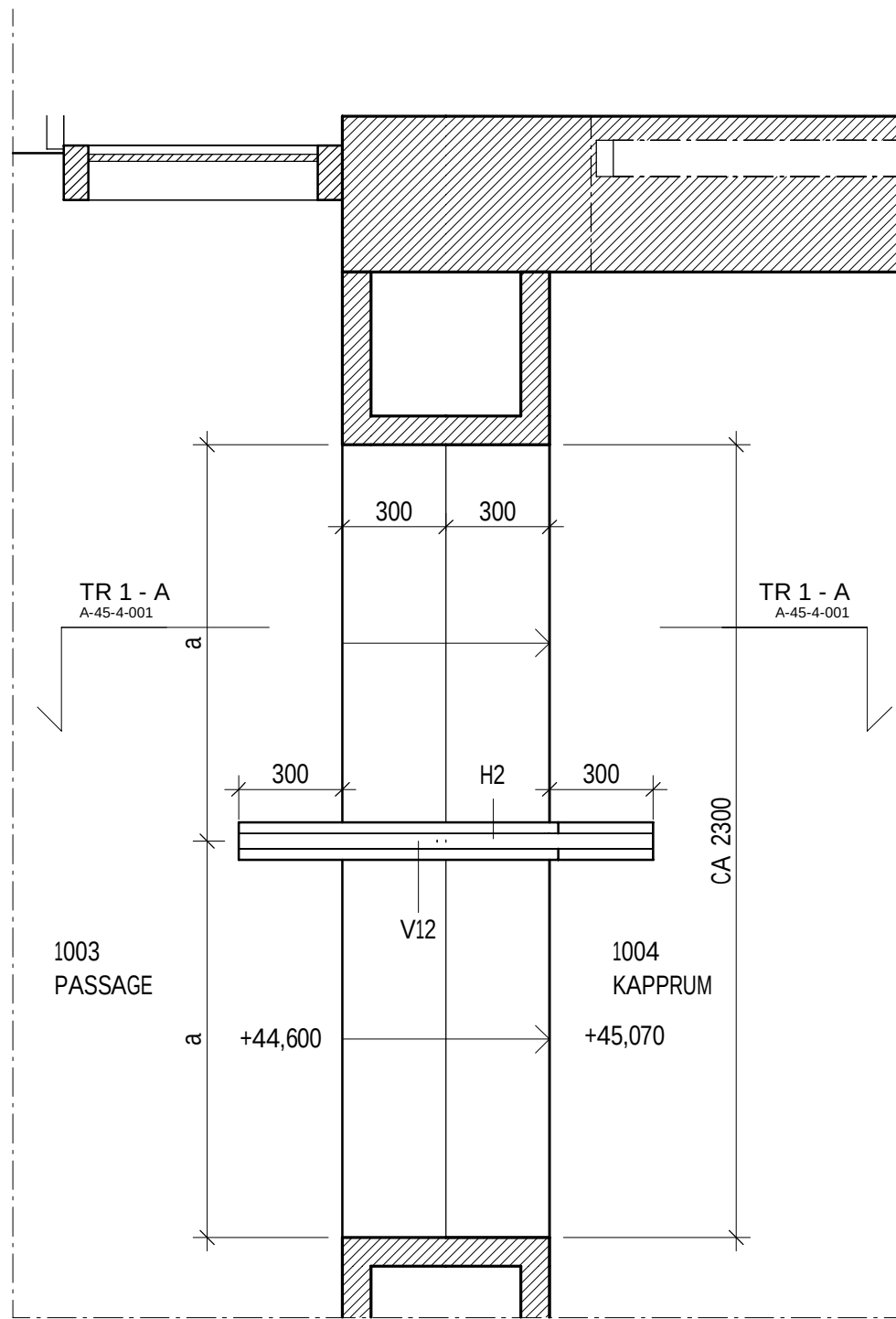
TRAPPA 1 - PLAN 1 : 20
