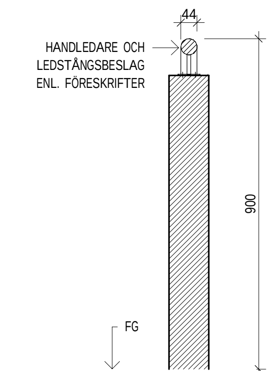
PRINCIPSEKTION HANDELDARE H2 1 : 10
