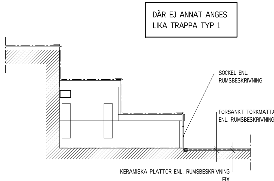
PRINCIPDETALJ TRAPPA TYP 2 1 : 10
