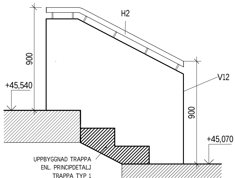
TRAPPA 2 - SEKTION A 1 : 20
