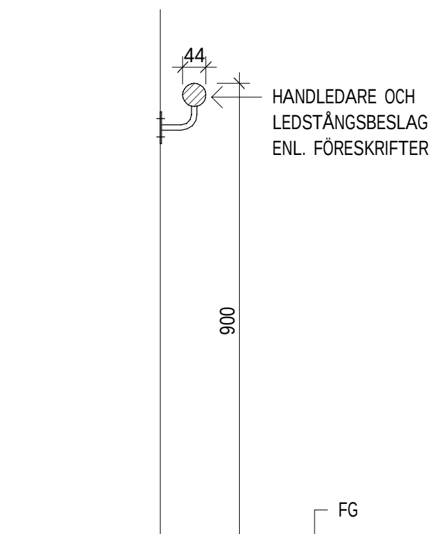
PRINCIP HANDELDARE H1 1 : 10
