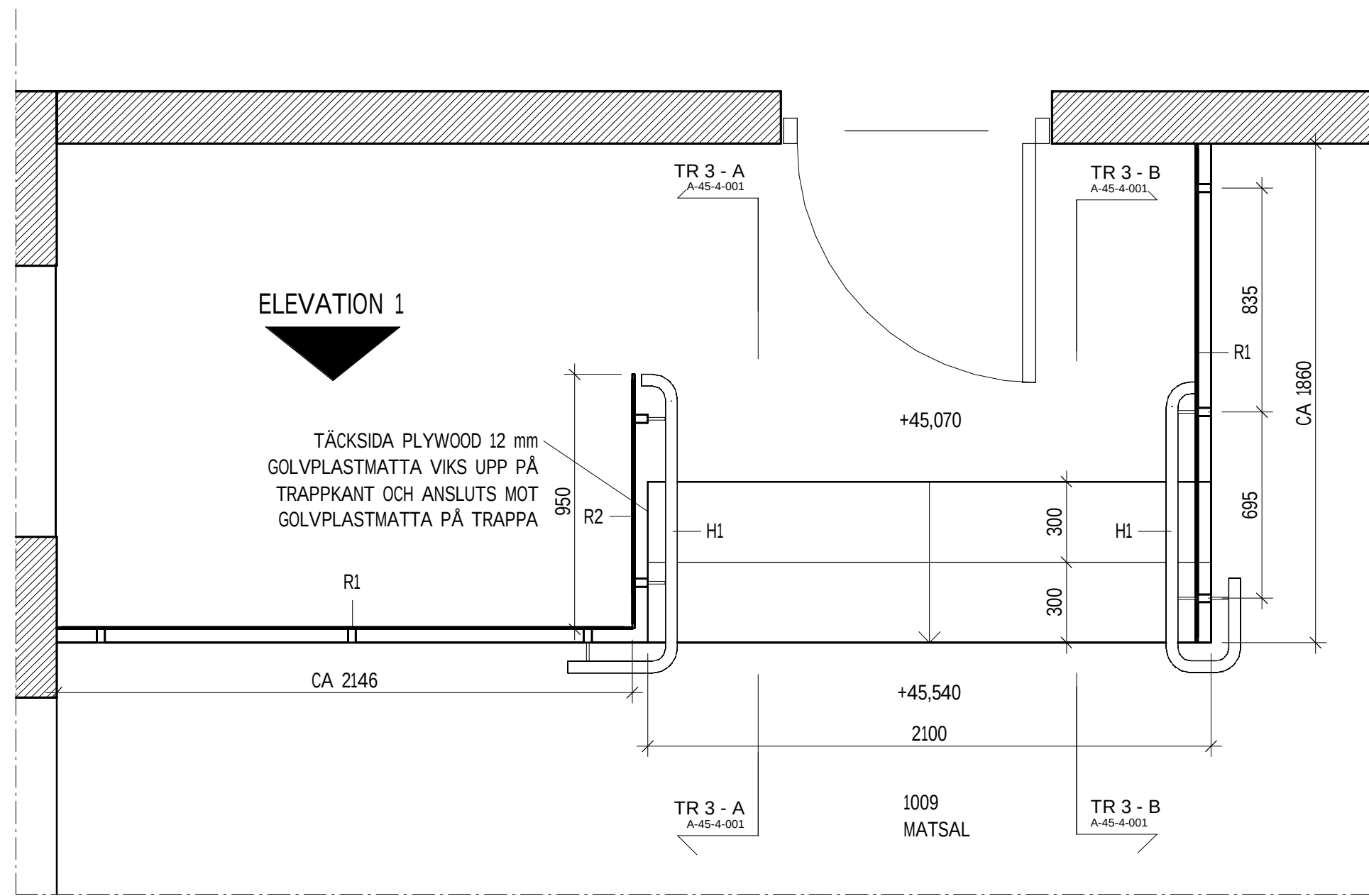
TRAPPA 3 - PLAN 1 : 20
