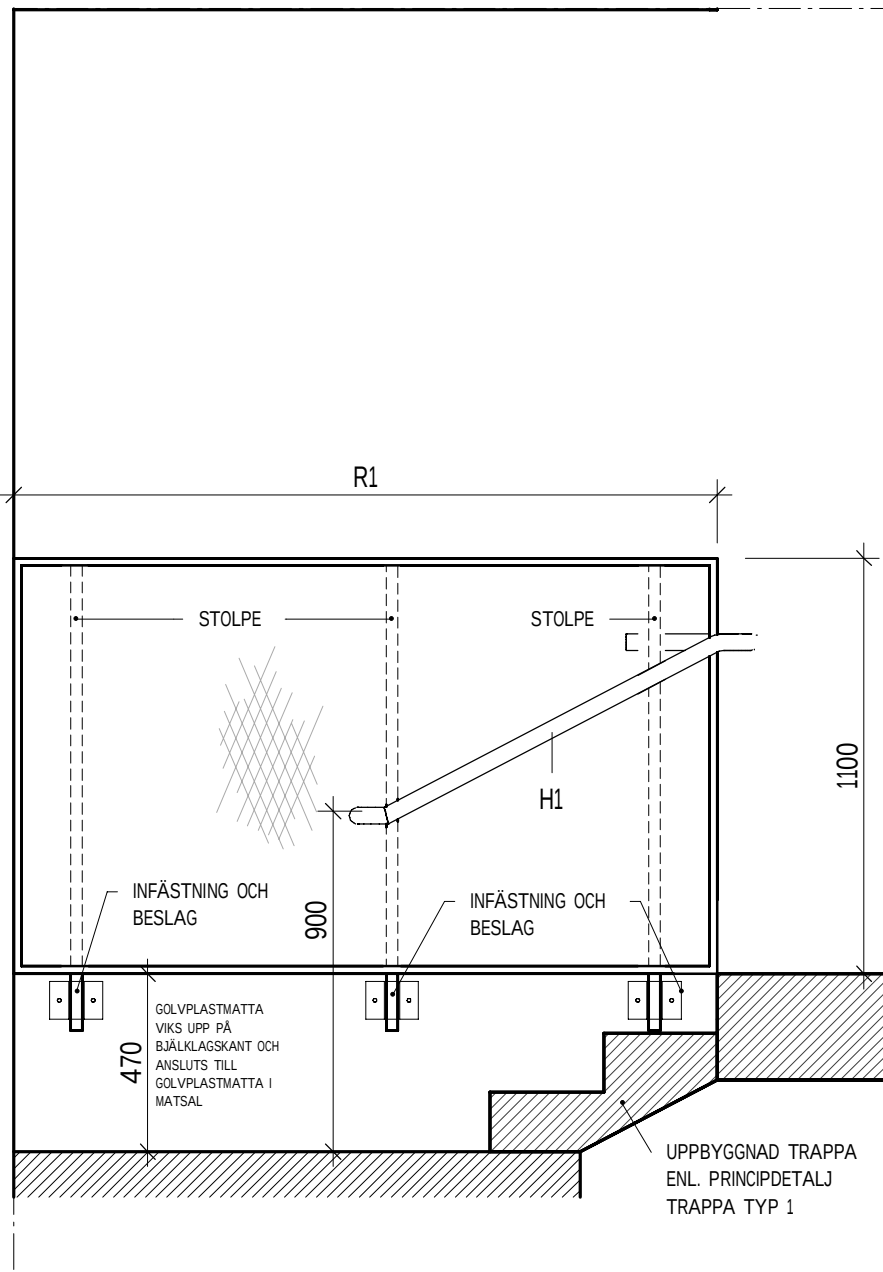
TRAPPA 3 - SEKTION B 1 : 20
