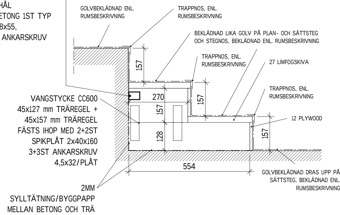
PRINCIPDETALJ TRAPPA TYP 1 1 : 10
